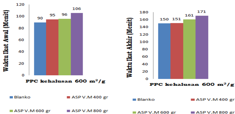
Gambar 1. Perpanjangan waktu ikat semen PPC kekehalusan 600 m 2 /g
